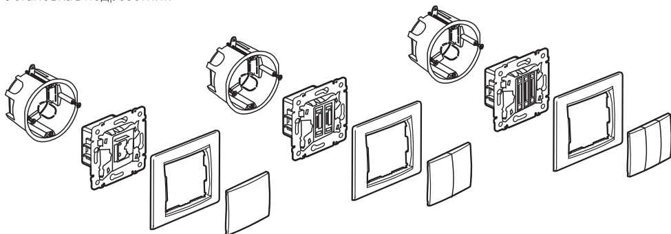
Установка в подрозетник
