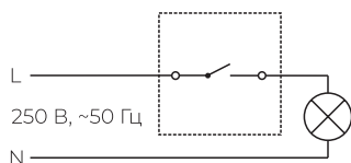
Одноклавишный выключатель
