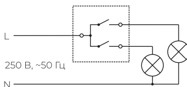
Двухклавишный выключатель
