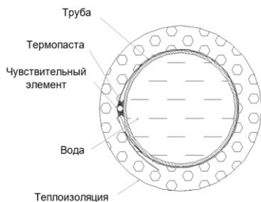
Схема установки датчика в бескорпусном исполнении
