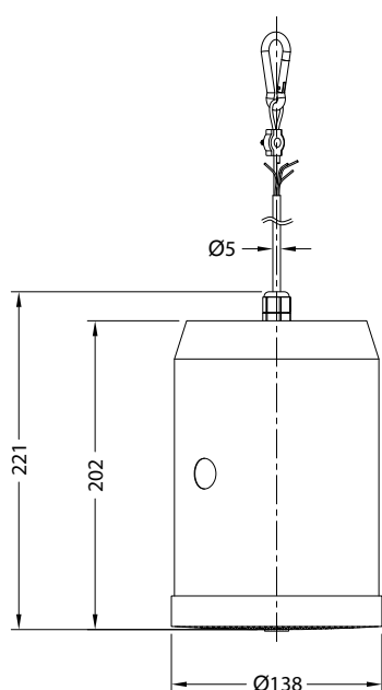
Вид сбоку
