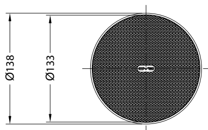
ВИД СНИЗУ / BOTTOM VIEW
