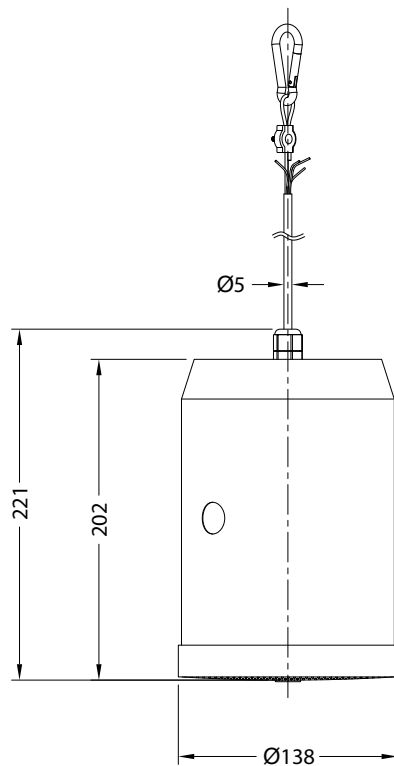
ВИД СБОКУ / SIDE VIEW
