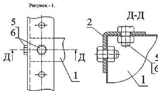
Крепление дополнительной полки без усиливающих уголков
