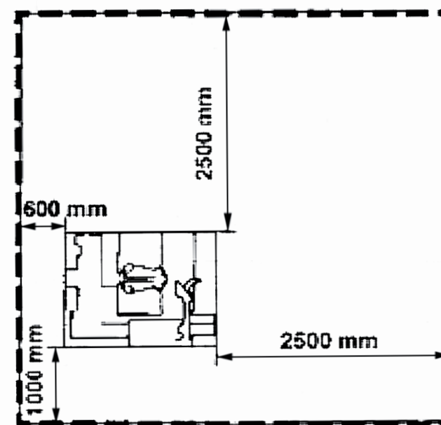
Рис. 2. Требования к расположению станка в помещении.
