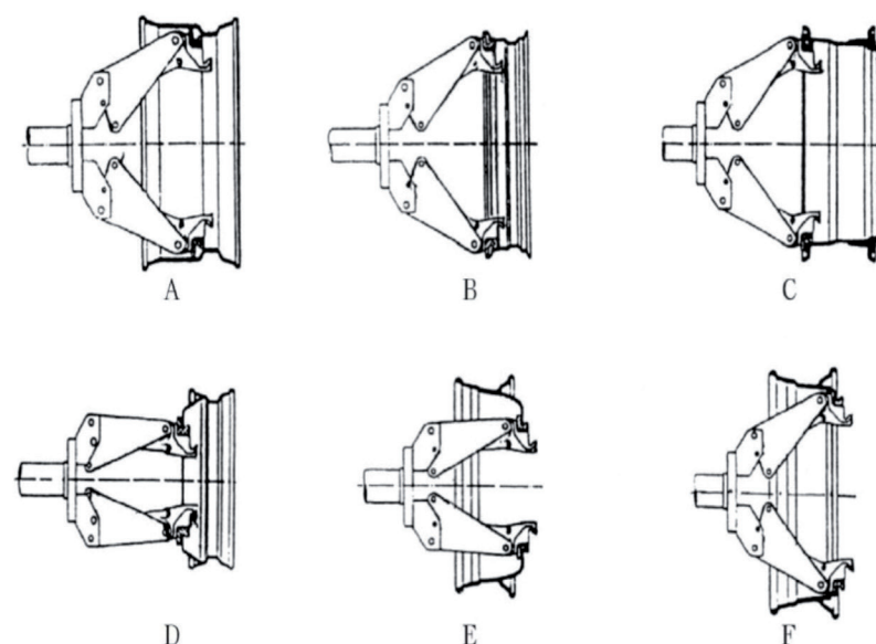
Рис. 7. Способы крепления ободов различных типов на шиномонтажном станке.
