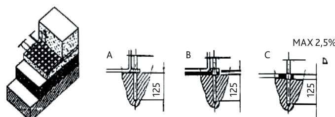
Рис. 3. Крепление рамы станка к полу анкерными болтами.
