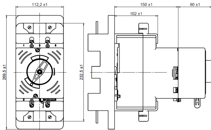
Рисунок Б.11 – Выключатель ВА57-35 с электромагнитным приводом на вытчной панели
