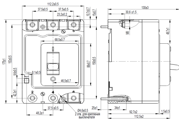
Рисунок Б.1 – Выключатель с зажимами для переднего присоединения
