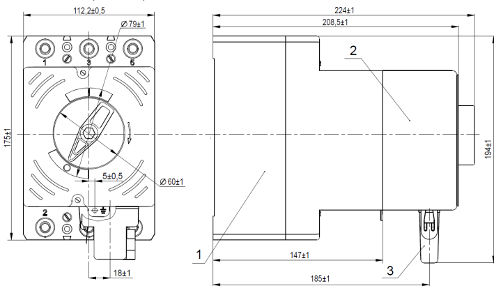
Рисунок Б.6 – Выключатель ВА57-35 с электромагнитным приводом 1 – выключатель; 2 – привод электромагнитный; 3 – соединитель типа РП10
