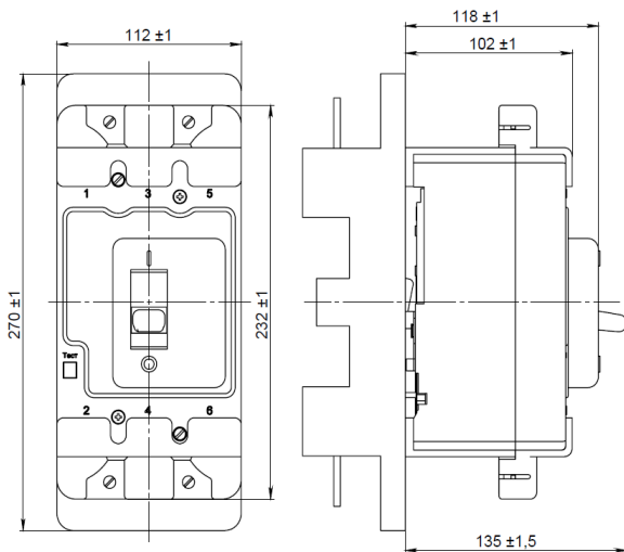
Рисунок Б.11 – Выключатель ВА57-35 с электромагнитным приводом на вытчной панели
