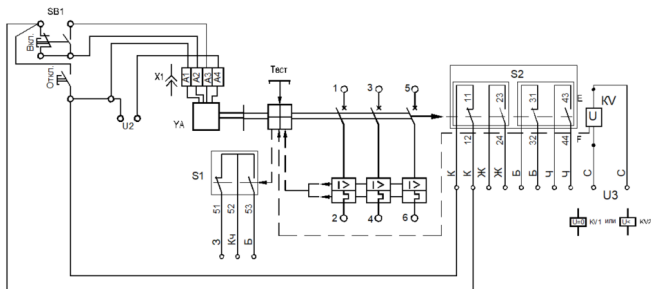
Рисунок Г.5 – Схема электрическая принципиальная выключателей выдвижного исполнения, с независимым расцепителем, вспомогательными контактами, вспомогательными контактами сигнализации автоматического отключения и электромагнитным приводом
