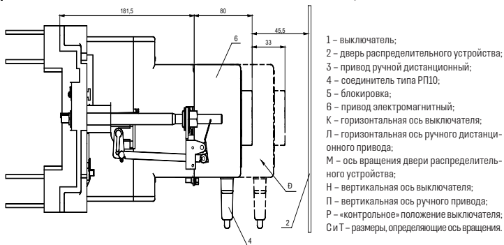
Рисунок Б.8 – Выключатель ВА57-35 выдвжного исполнения с электромагнитным приводом
