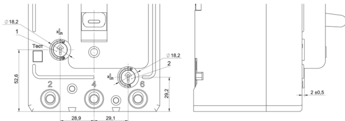
Рисунок 1 – Выключатель с регулируемыми максимальными расцепителями
