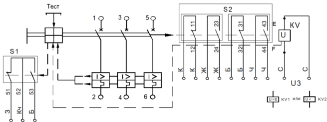
Рисунок Г.3 – Схема электрическая принципиальная выключателей стационарного исполнения, с нулевым или минимальным расцепителем напряжения, вспомогательными контактами сигнализации автоматического отключения и вспомогательными контактами
