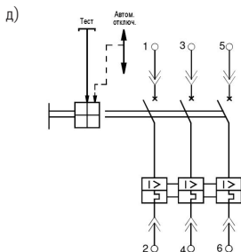
Рисунок Г.2 – Схема электрическая принципиальная выключателя стационарного исполнения, переменного тока трех-полюсного исполнения с независимым расцепителем и вспомогательными контактами
