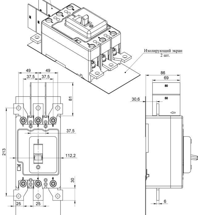
Рисунок Д.26 – Присоединение с расширительными выводами, межполюсными перегородками и изолирующими экранами Расширительные выводы рекомендуется использовать совместно с изолирующими экранами.
