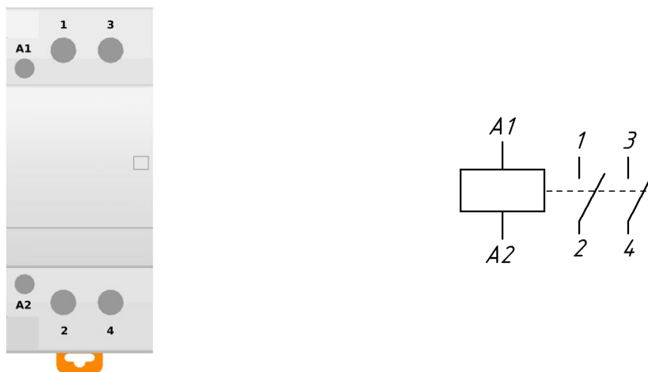
Рисунок А.1 – Принципиальная электрическая схема и расположение контактов
