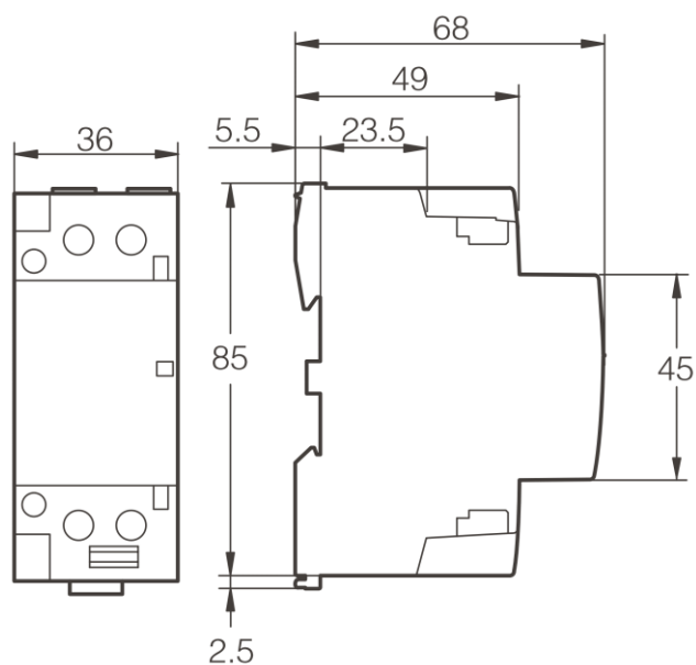
Рисунок А.2 – Габаритные размеры
