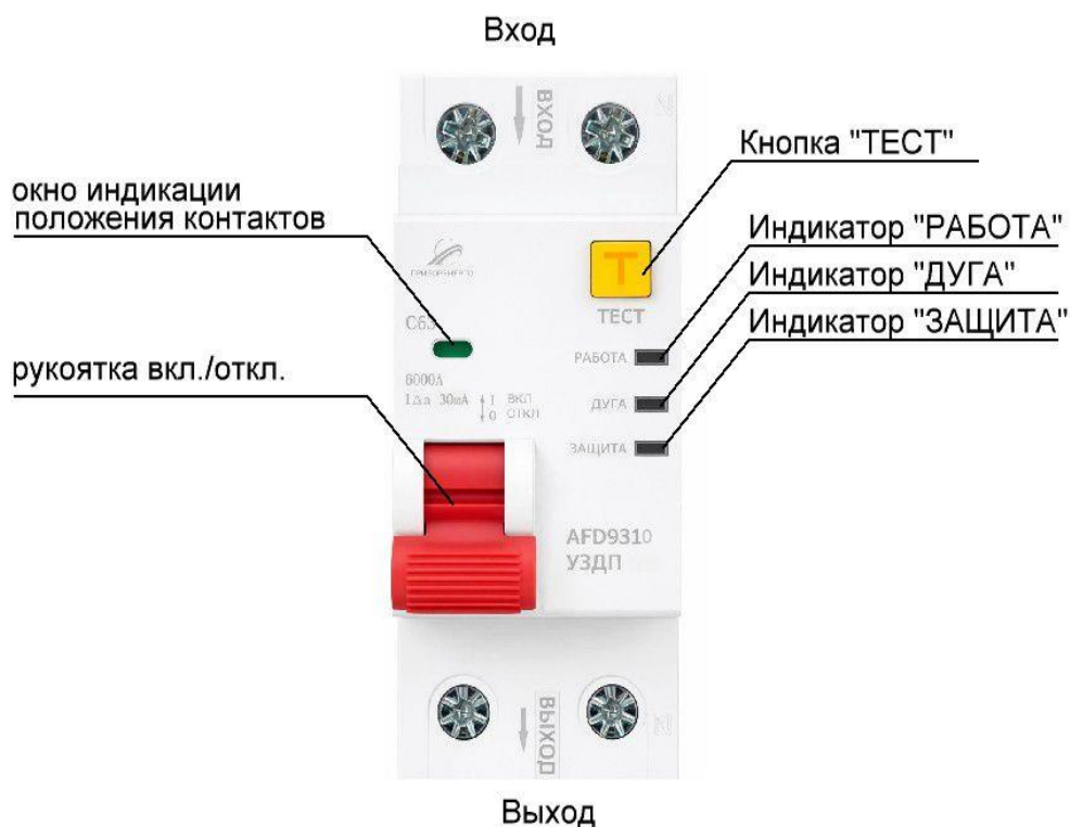
Рисунок 1 – Органы индикации и управления УЗДП AFD9317
