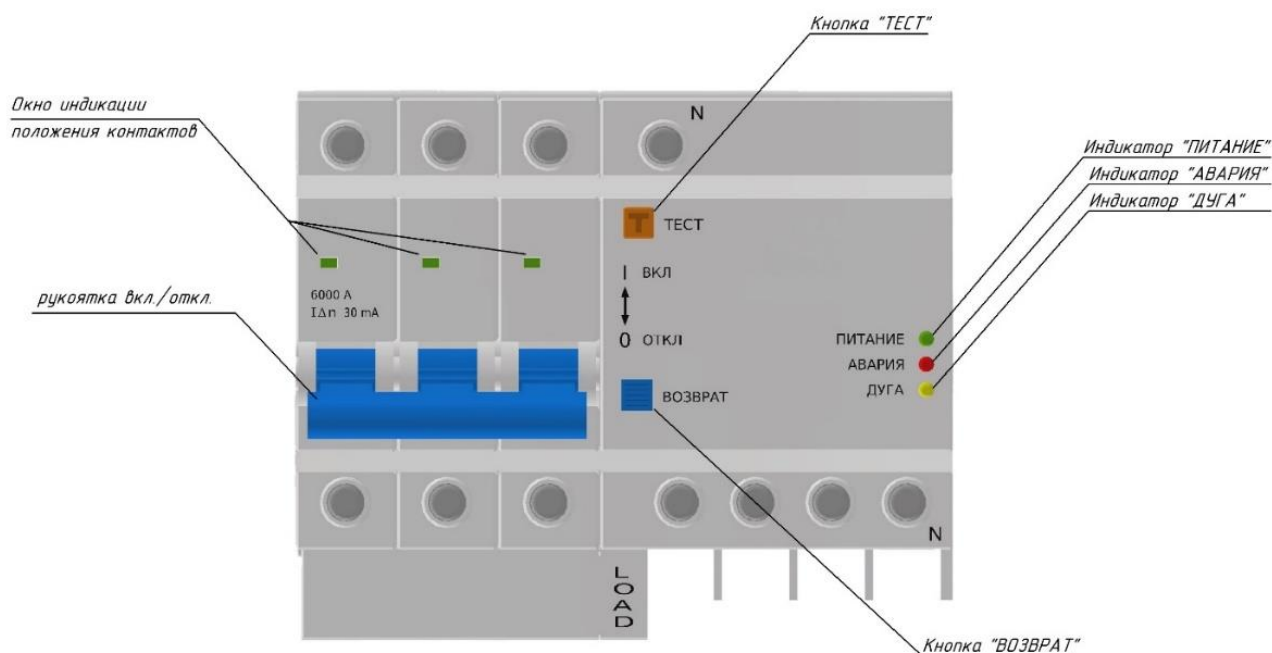
Рисунок 1 – Органы индикации и управления УЗДП AFD9413
