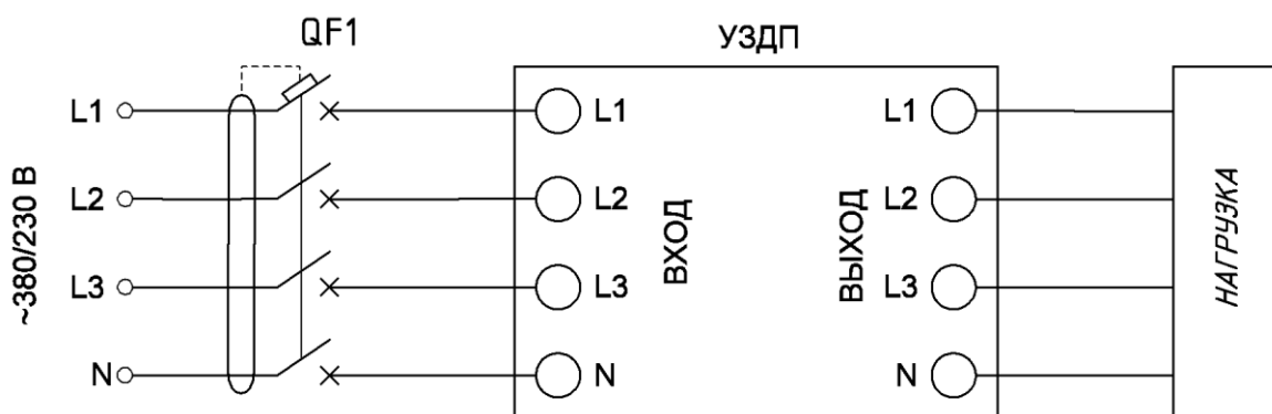
Рисунок Б.3 – Схема подключения УЗДП AFD9413 с устройством защитного отключения (УЗО)
