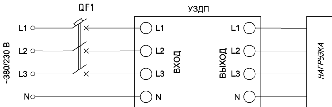
Рисунок Б.1 – Схема подключения УЗДП AFD9413 с автоматическим выключателем (АВ)
