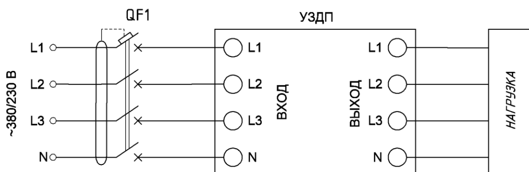
Рисунок Б.2 – Схема подключения УЗДП AFD9413 с дифференциальным автоматом (ДА)
