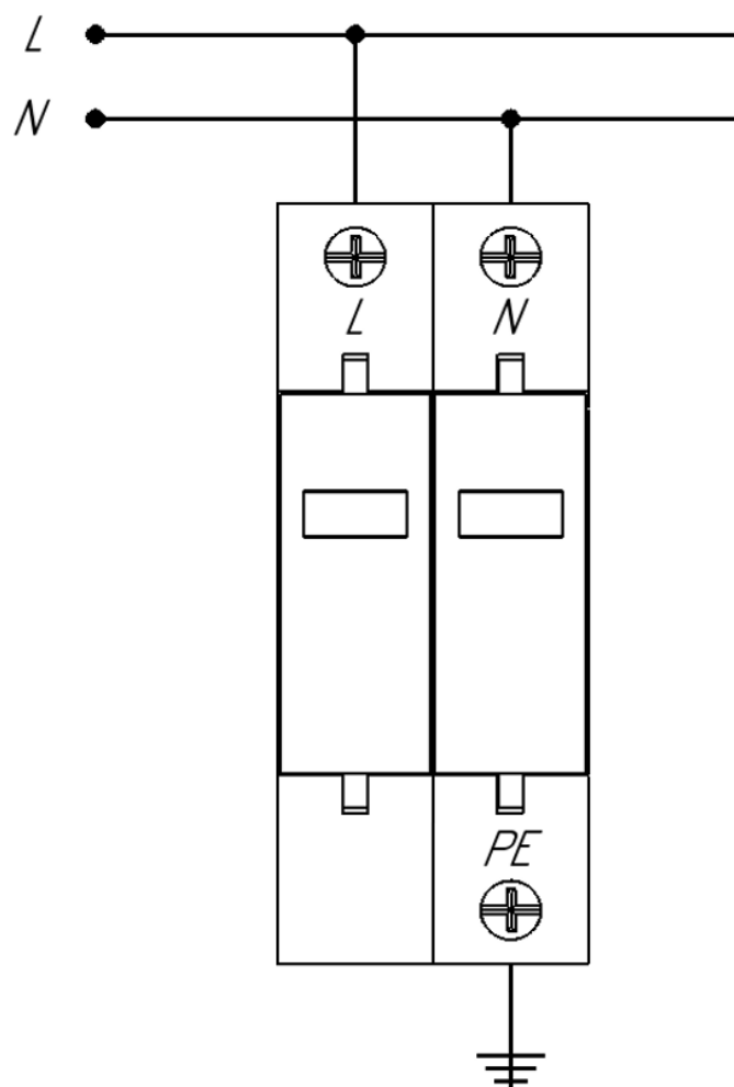
Рисунок Б.1 – Схема УЗИП ОПС-44Е-2PN 1+2 класса
