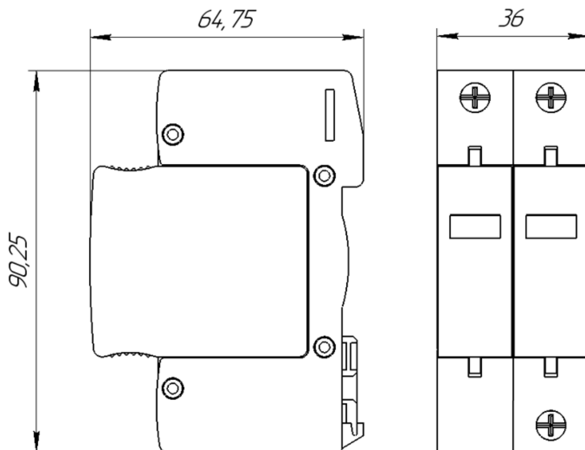
Рисунок А.1 – Габаритные размеры
