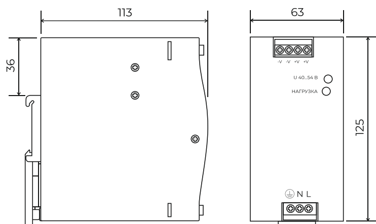
Размеры
