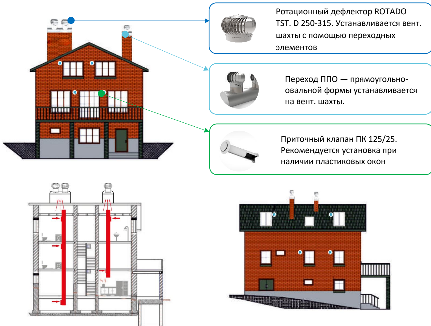
Рис. 8. Примеры установки ротационного дефлектора на переход ППО
