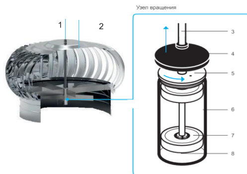
Рис. 11. Схема узла вращения.
