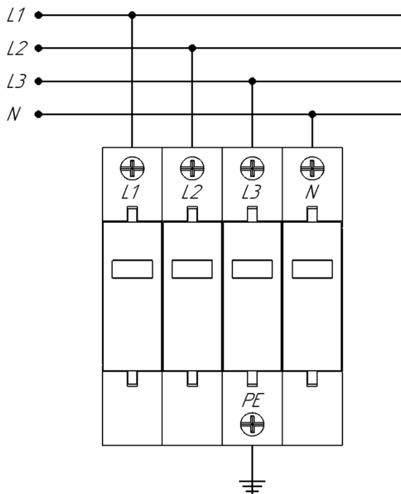
Рисунок Б.1 – Схема УЗИП ОПС-44Е-4РN 1+2 класса
