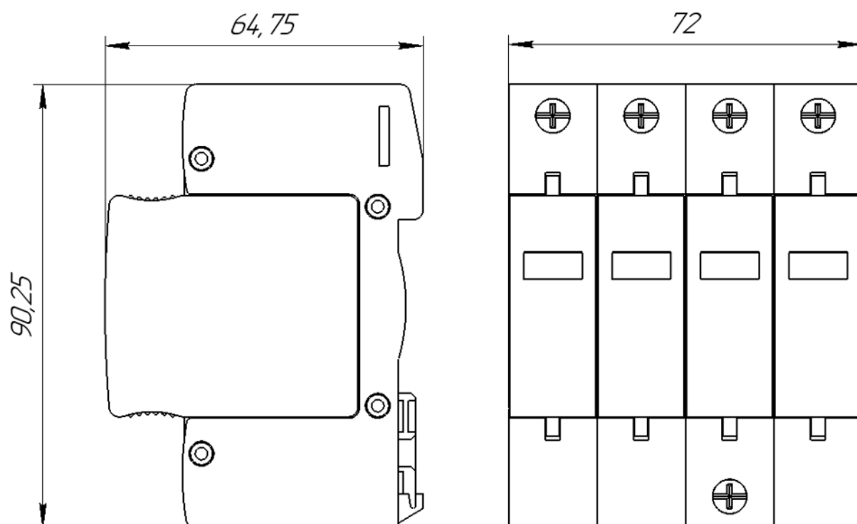
Рисунок А.1 – Габаритные размеры
