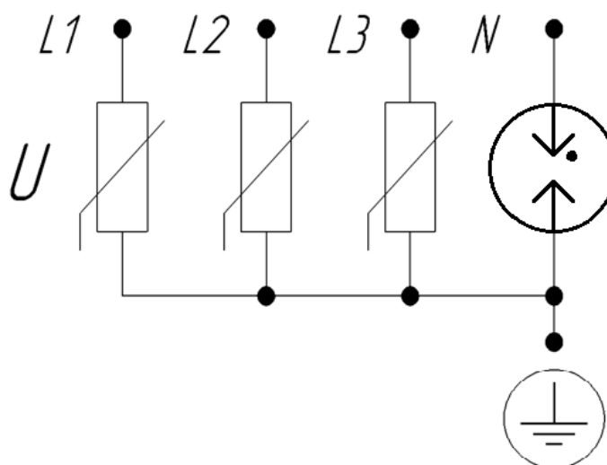
Рисунок Б.2 – Схема электрическая принципиальная
