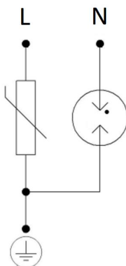
Рисунок Б.2 – Схема электрическая принципиальная
