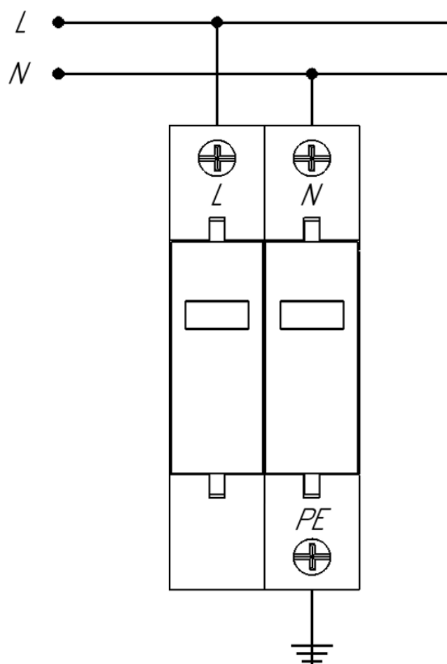
Рисунок Б.1 – Схема УЗИП ОПС-34Е-2РN 1+2 класса
