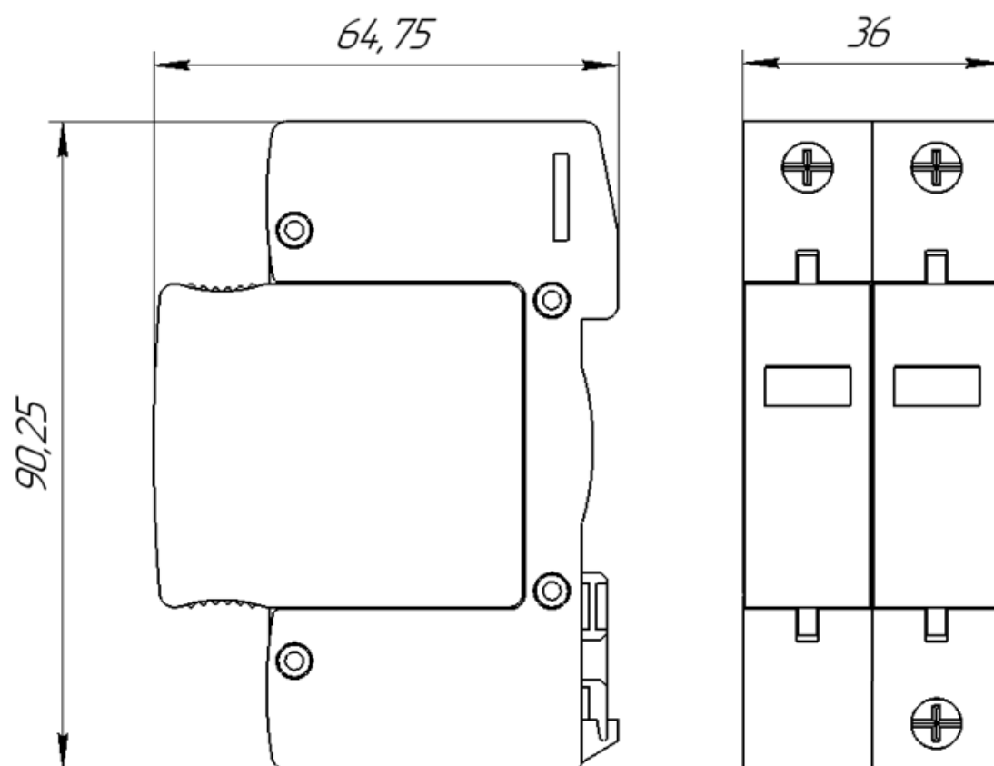
Рисунок А.1 – Габаритные размеры
