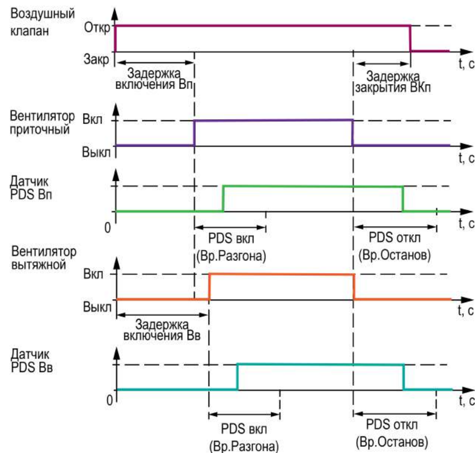
Рисунок 10.8 – Управление вентиляторами
