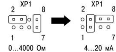
Рисунок 10.5 – Изменение конфигурации перемычек
