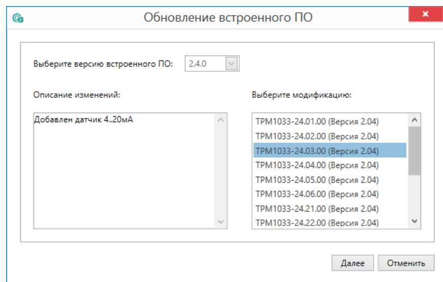
Рисунок 11.7 – Выбор алгоритма
