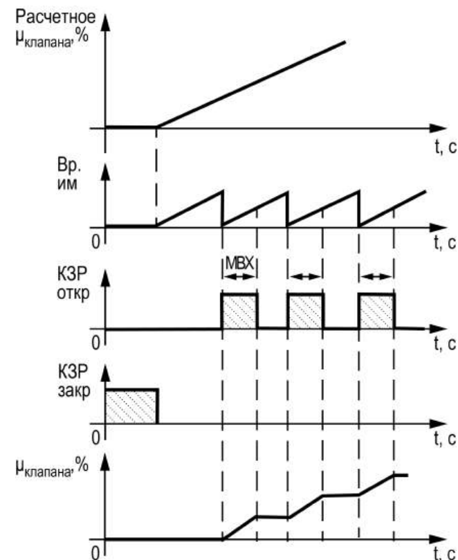
Рисунок 10.1 – Работа КЗР
