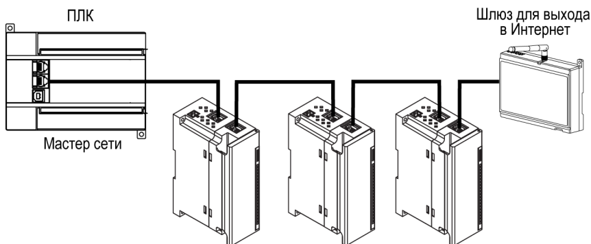
Рисунок 5.13 – Подключение по схеме «Цепочка»
