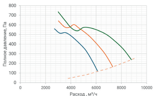
Графики аэродинамических характеристик осевых вентиляторов WEPS-K
