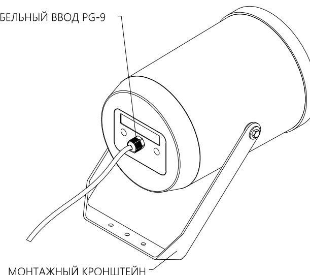
МОНТАЖНЫЙ КРОНШТЕЙН
