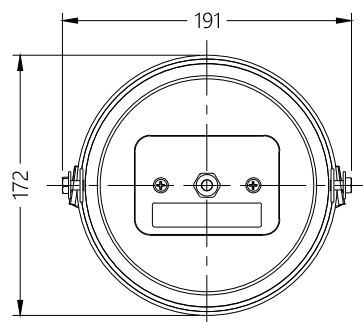
ВИД СЗАДИ / REAR VIEW
