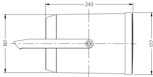
ВИД СБОКУ / SIDE VIEW
