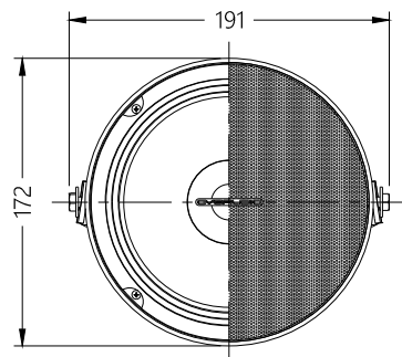
ВИД СПЕРЕДИ / FRONT VIEW
