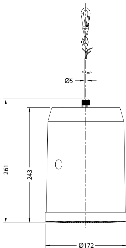
ВИД СБОКУ / SIDE VIEW
