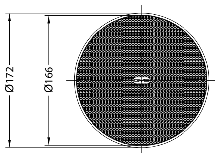
ВИД СНИЗУ / BOTTOM VIEW
