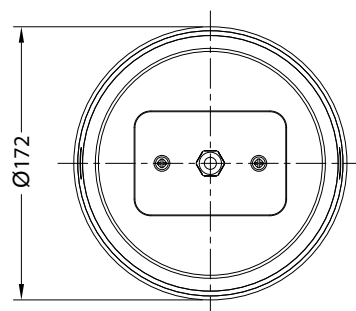
ВИД СВЕРХУ / TOP VIEW
