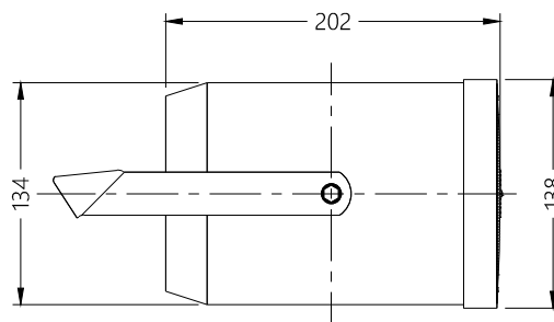
ВИД СБОКУ / SIDE VIEW
