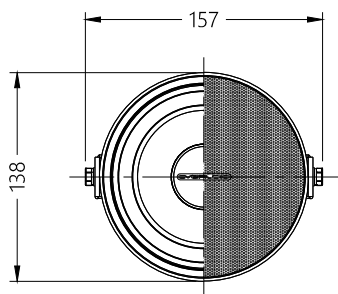
ВИД СПЕРЕДИ / FRONT VIEW
