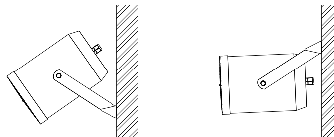
СПОСОБ МОНТАЖА НА СТЕНУ / WALL MOUNTING METHOD
