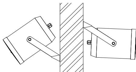
Способ монтажа на стену
