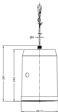
Вид сбоку
