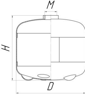
Рисунок 2 – Общий вид баллона
