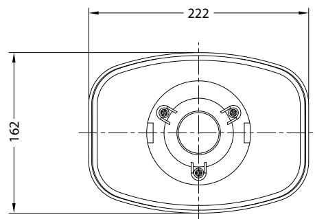
ВИД СПЕРЕДИ / FRONT VIEW
