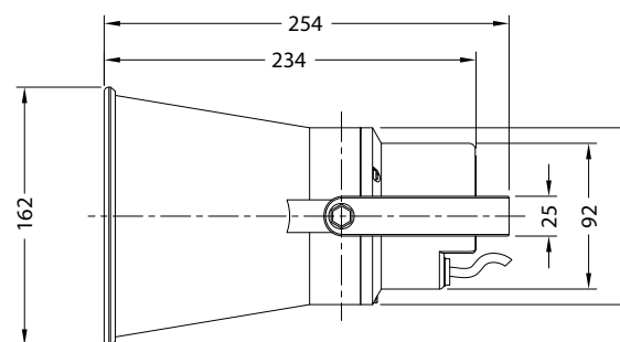
ВИД СБОКУ / SIDE VIEW
