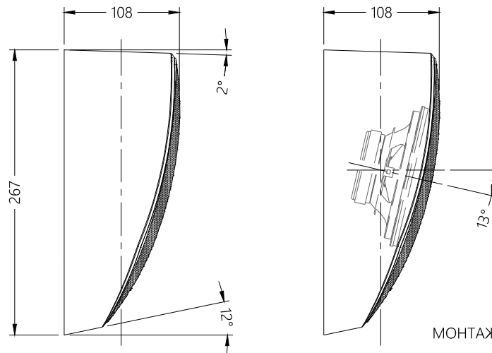
ШАБЛОН ЧЕРТЕЖА ДЛЯ УСТАНОВКИ АКУСТИЧЕСКОЙ СИСТЕМЫ / DRAWING TEMPLATE FOR INSTALLING A SPEAKER SYSTEM
