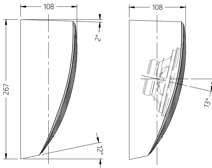
Вид сбоку
