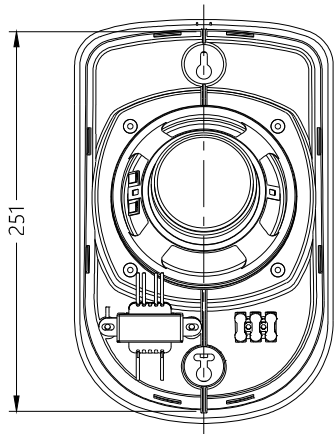
ВИД СВЕРХУ / TOP VIEW
