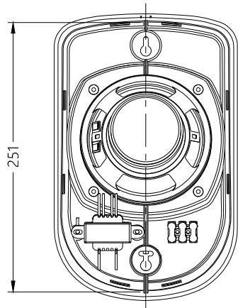
ВИД СВЕРХУ / TOP VIEW
