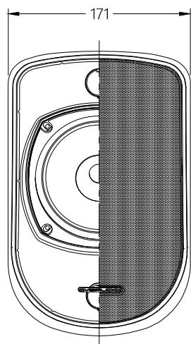
ВИД СПЕРЕДИ / FRONT VIEW
