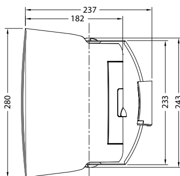
ВИД СВЕРХУ / TOP VIEW
