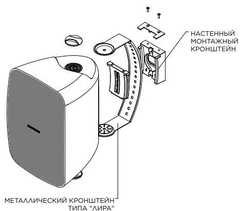
МОНТАЖНЫЙ КРОНШТЕЙН / MOUNTING BRACKET
