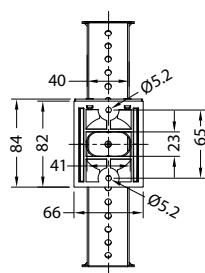
ВИД СЗАДИ / REAR VIEW
