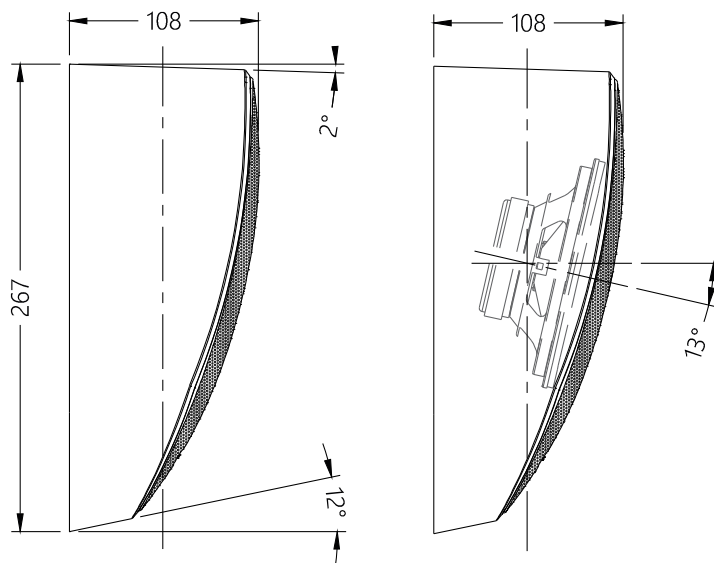
Вид сбоку
