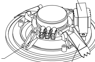
КЛЕММА САМОЗАЖИМНАЯ СН-3
