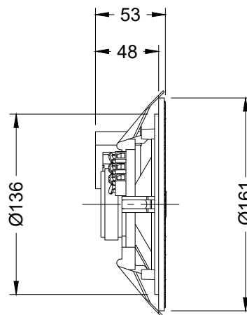
ВИД СБОКУ / SIDE VIEW
