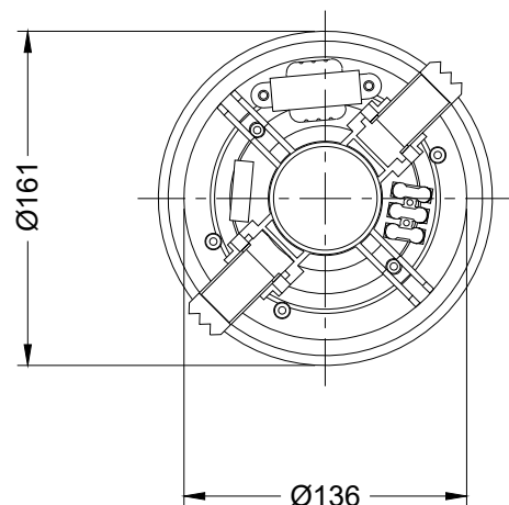
ВИД СВЕРХУ / TOP VIEW
