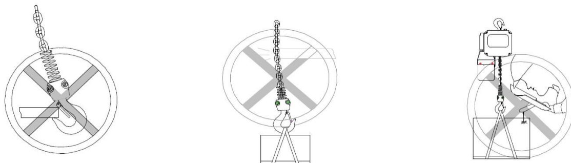
Рисунок 7. Правила использования тали.
