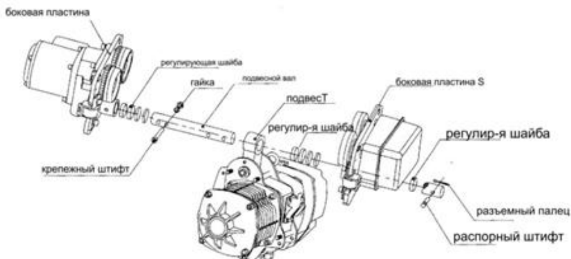
Рисунок 11. Таль с тележкой.
