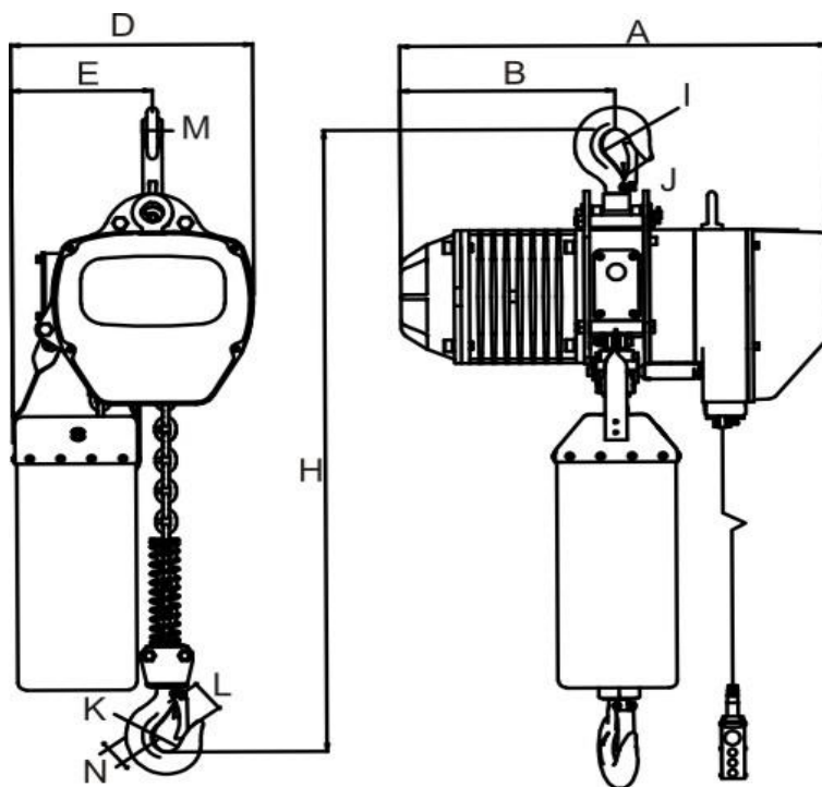
Рисунок 4. Таль электрическая ННВ.
