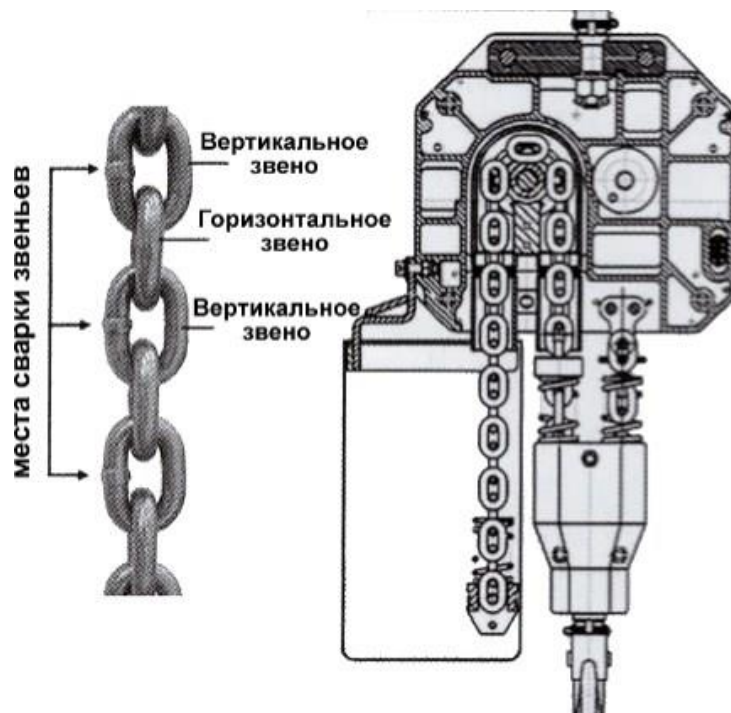
Рисунок 15 Звенья цепи.
