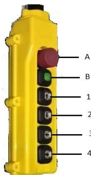
Рисунок 5 Пульт управления
