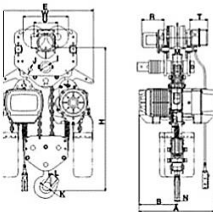
Рисунок 3. Таль электрическая цепная ННВ4(Т).
