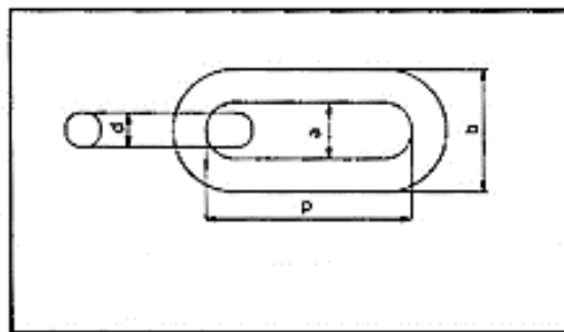
Рисунок 13. Размеры цепи.
