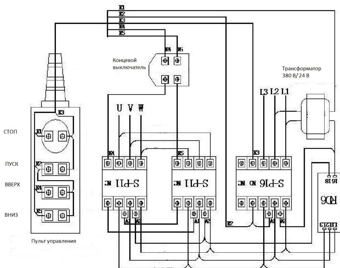
RD 6 блок контроля фаз
