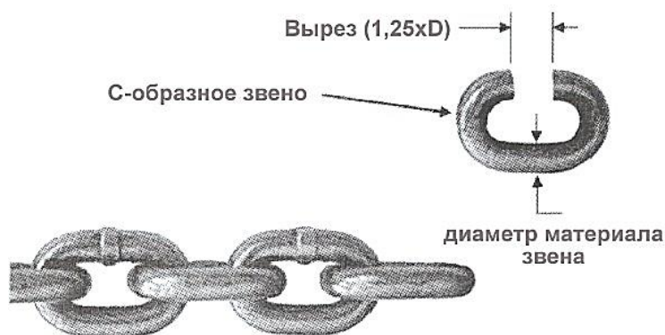
Рисунок 14. С-образное звено.
