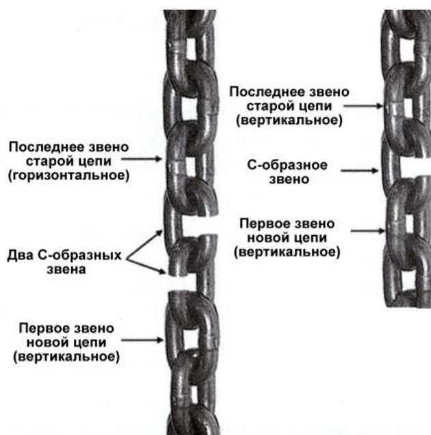
Рисунок 16 Соединение цепей.
