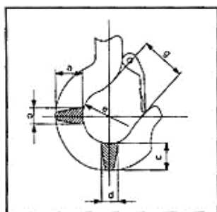
Рисунок 17. Размер крюк.
