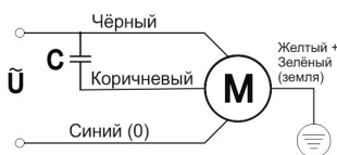
Схема подключения
