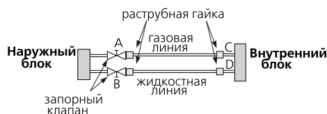
A: Запорный клапан низкого давления B: Запорный клапан высокого давления C и D: Концы трубопроводов.
