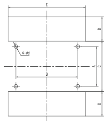
Рисунок 2. Установочные размеры выкатного присоединения KA-330E
