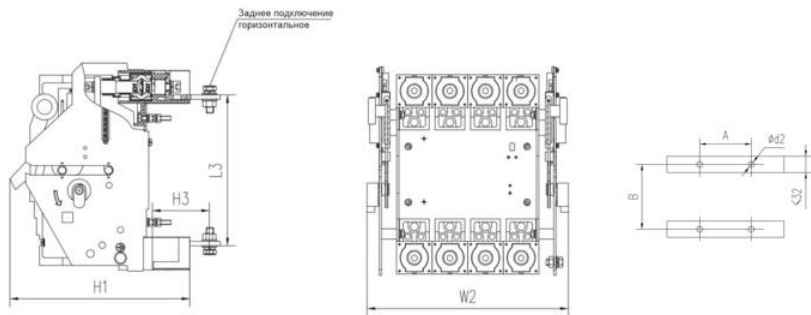
Рисунок 1. Габаритные и установочные размеры выкатного присоединения KA-330E
