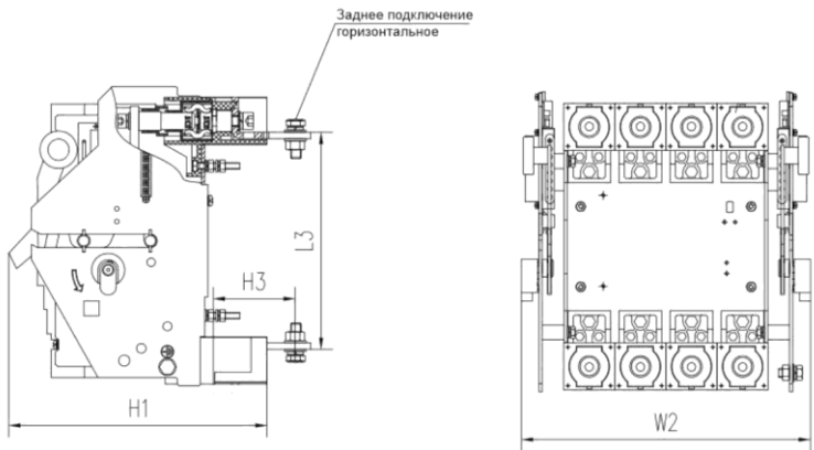
Рисунок 1. Габаритные размеры выкатного присоединения KA-300
