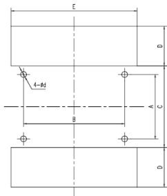
Рисунок 2. Установочные размеры выкатного присоединения KA-300
