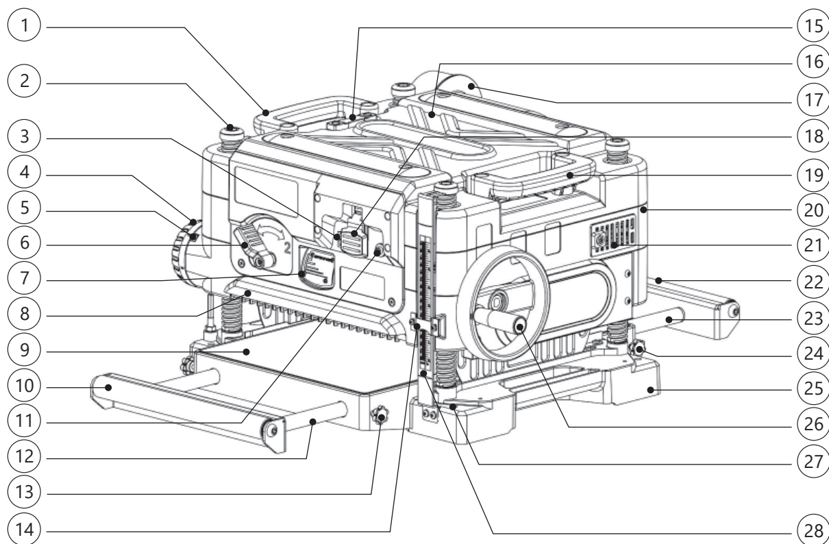
Рисунок 1. Основные элементы станка BELMASH P2000D и BELMASH P2000DH.
