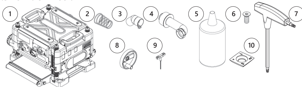
Рисунок 2. Комплектация станка BELMASH P2000D и BELMASH P2000DH.
