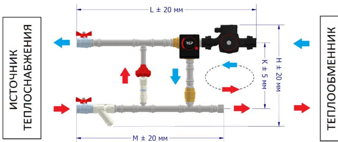
Схема смесительных узлов обратной конфигурации с байпасом
