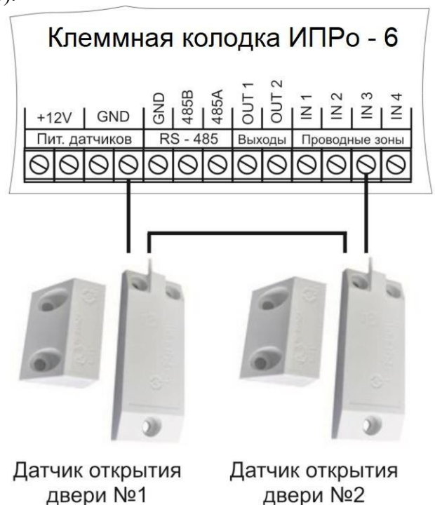
Подключение 2-х датчиков
