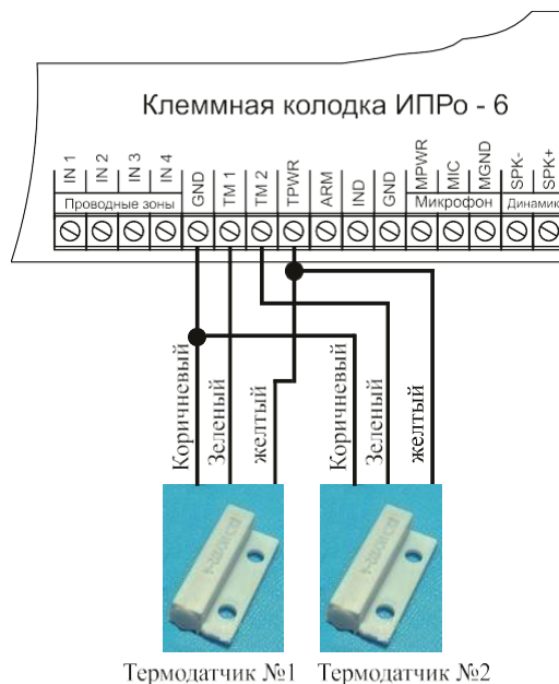
Подключения 2-х датчиков
