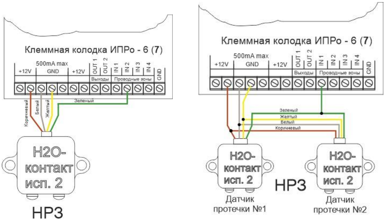
Подключение 1 датчика
