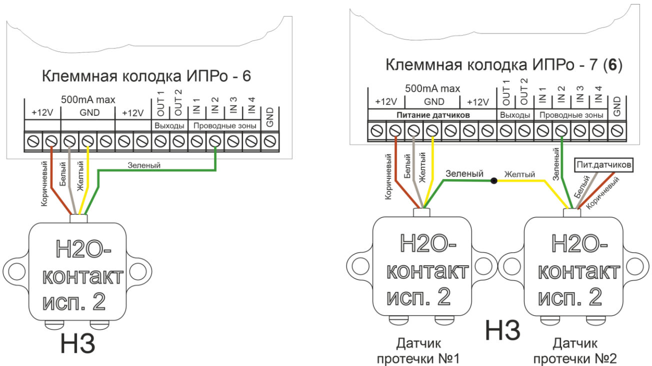
Подключение 1 датчика
