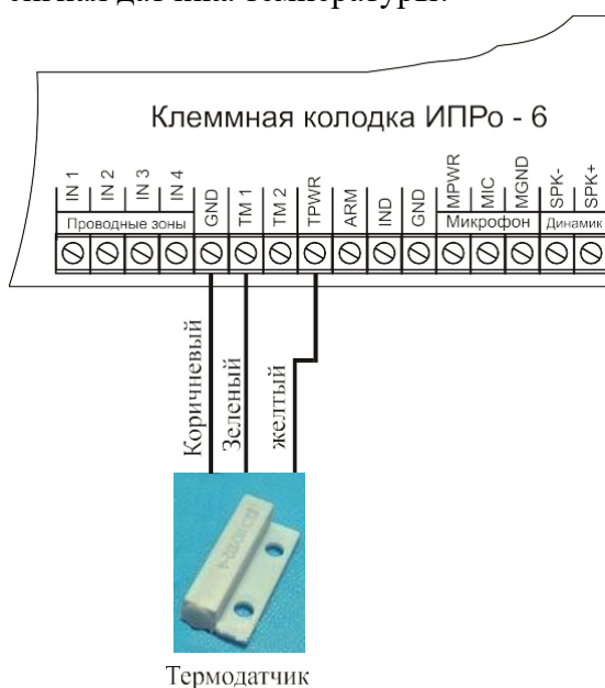
Подключение одного датчика
