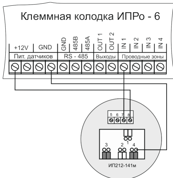
Подключение 1 датчика
