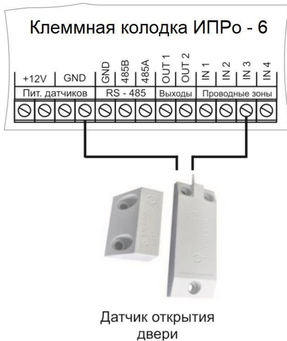
Подключение 1 датчика
