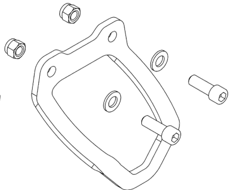
рис. 3 Крепление анкерной точки на металлическое основание
