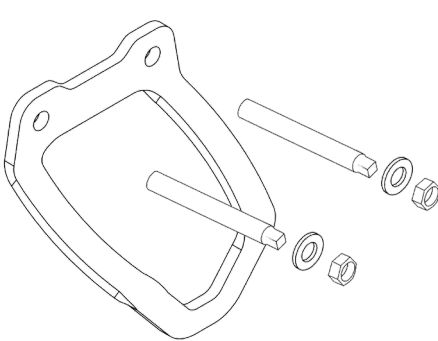
рис. 2 Крепление анкерной точки в бетон / кирпич
