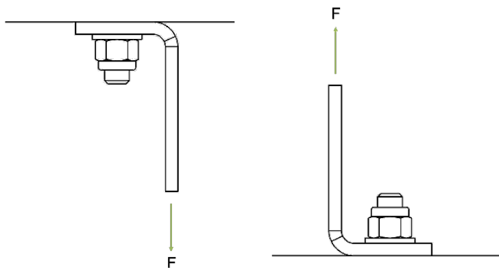
рис. 1 Пространственное положение крепления анкерной точки
