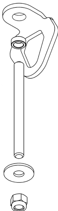
рис. 2 Крепление анкерной точки в бетон / кирпич
