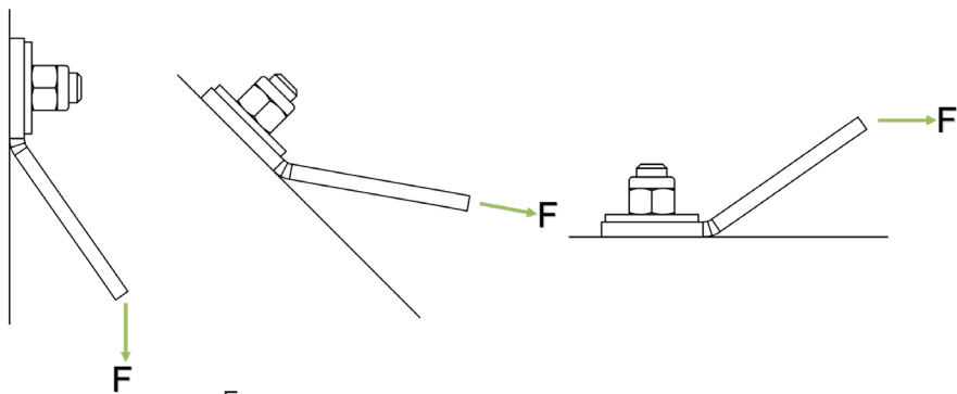
рис. 1 Пространственное положение крепления анкерной точки
