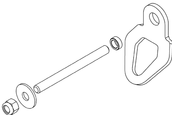
рис. 2 Крепление анкерной точки в бетон / кирпич
