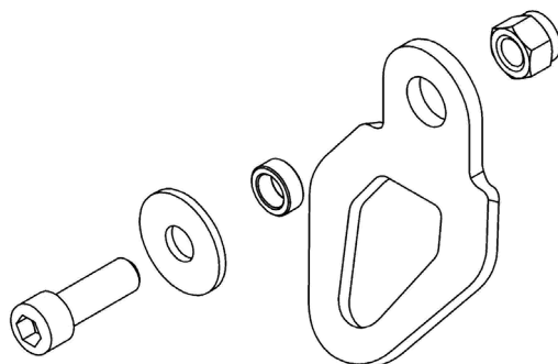
рис. 3 Крепление анкерной точки на металлическое основание
