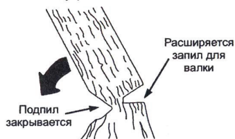
Недопил поддерживает дерево и помогает управлять валкой.
