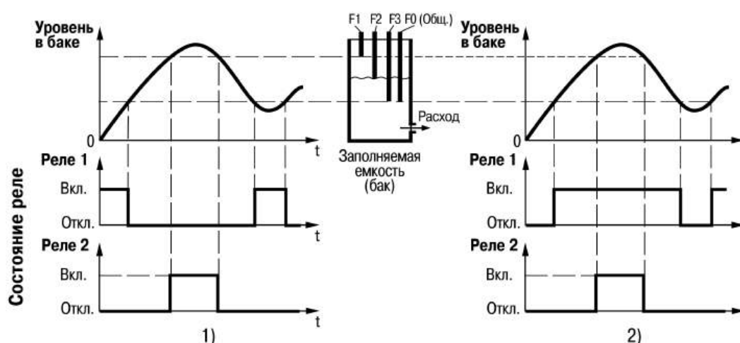
Рисунок 9.3 – Графики работы прибора: 1) заполнение, 2) осушение
