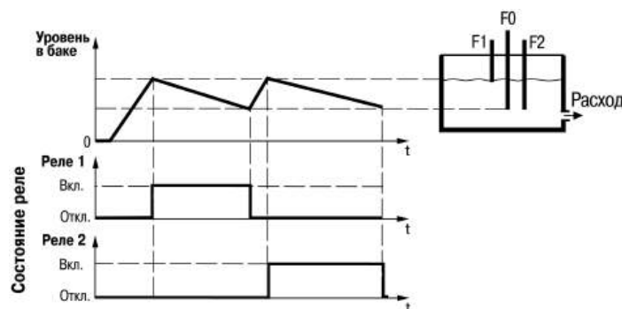
Рисунок 9.13 – Графики работы прибора
