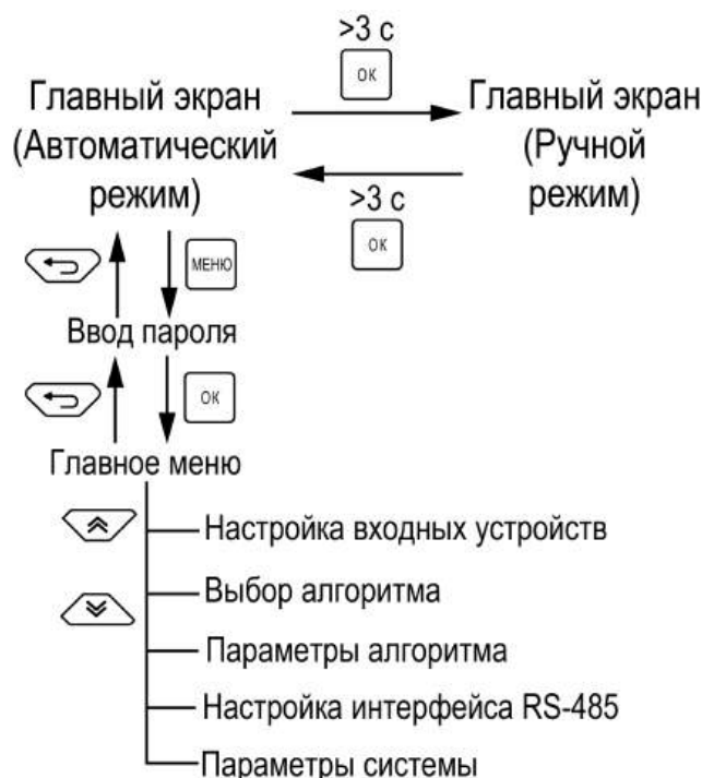
Рисунок 8.1 – Меню
