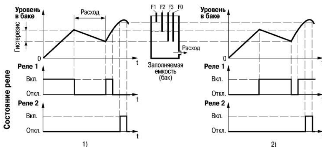
Рисунок 9.2 – Графики работы прибора: 1) заполнение, 2) осушение
