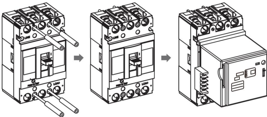
Рисунок 3. Схема установки привода моторного для BA-333E, BA-335E, BA-336E
