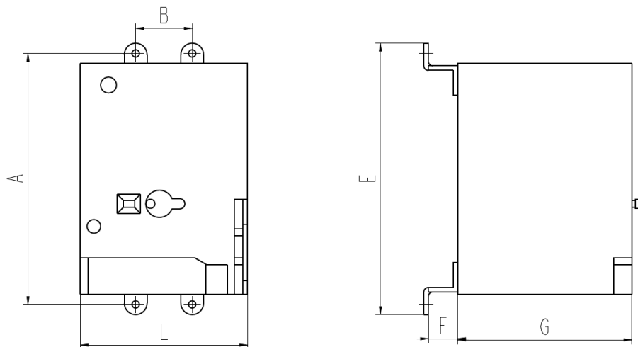
Рисунок 2. Габаритные и установочные размеры привода моторного МП-333Е, МП-335Е, МП-336Е
