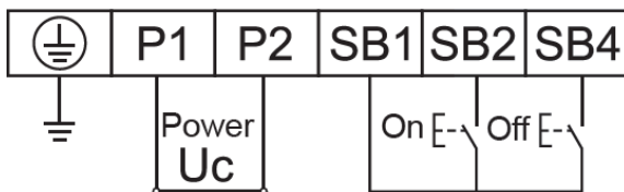
Рисунок 1. Схема электрических соединений
