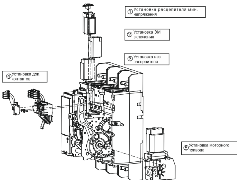
Рисунок 3. Схема установки привода моторного для BA-338E
