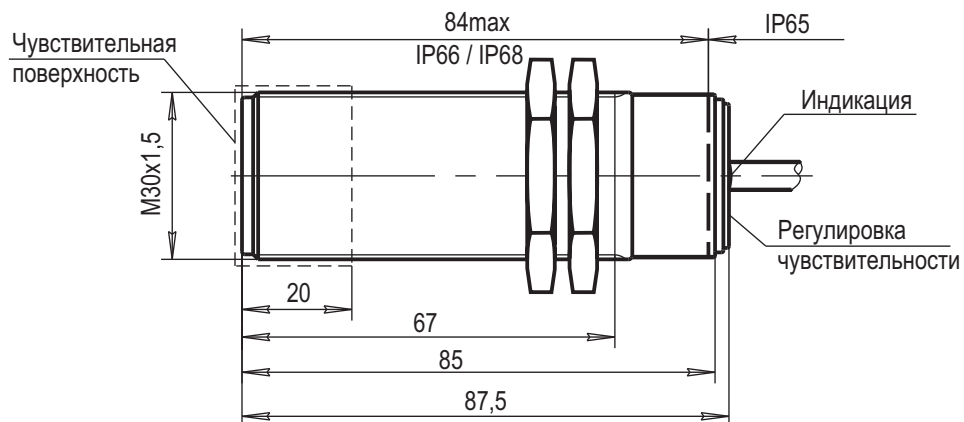
Габаритный чертеж
