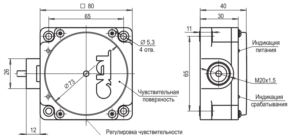
Габаритный чертеж
