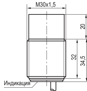
Габаритный чертеж
