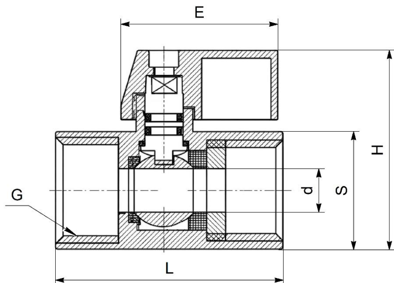
Рисунок 4 – Размеры изделия
