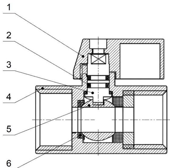
Рисунок 3 – Составные части изделия
